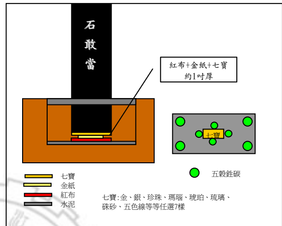
圖 3-5-3 石敢當安豎示意圖(一)
